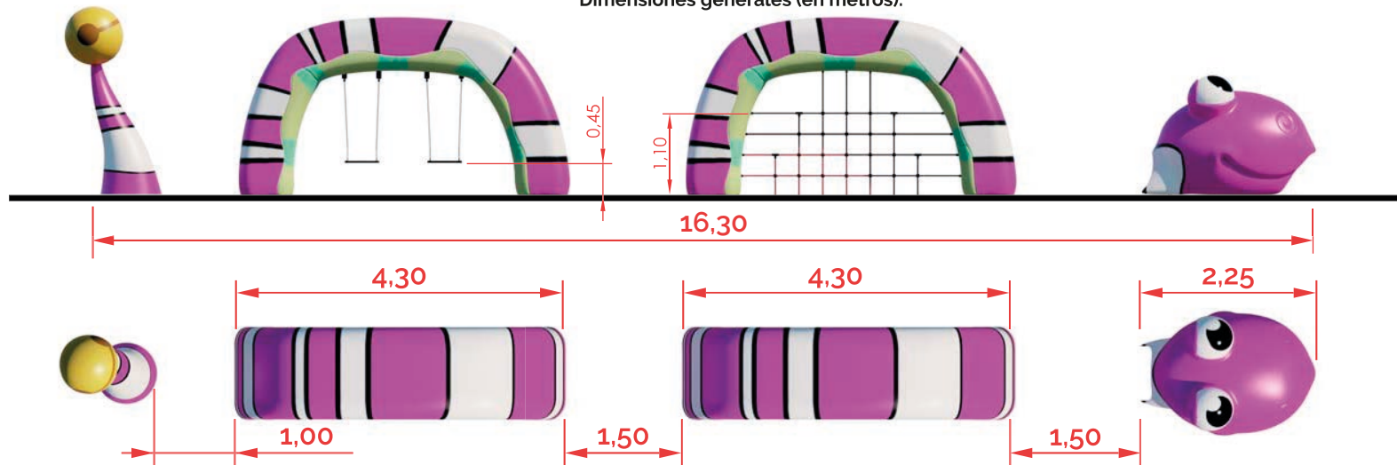
Dimensiones generales (en metros).
