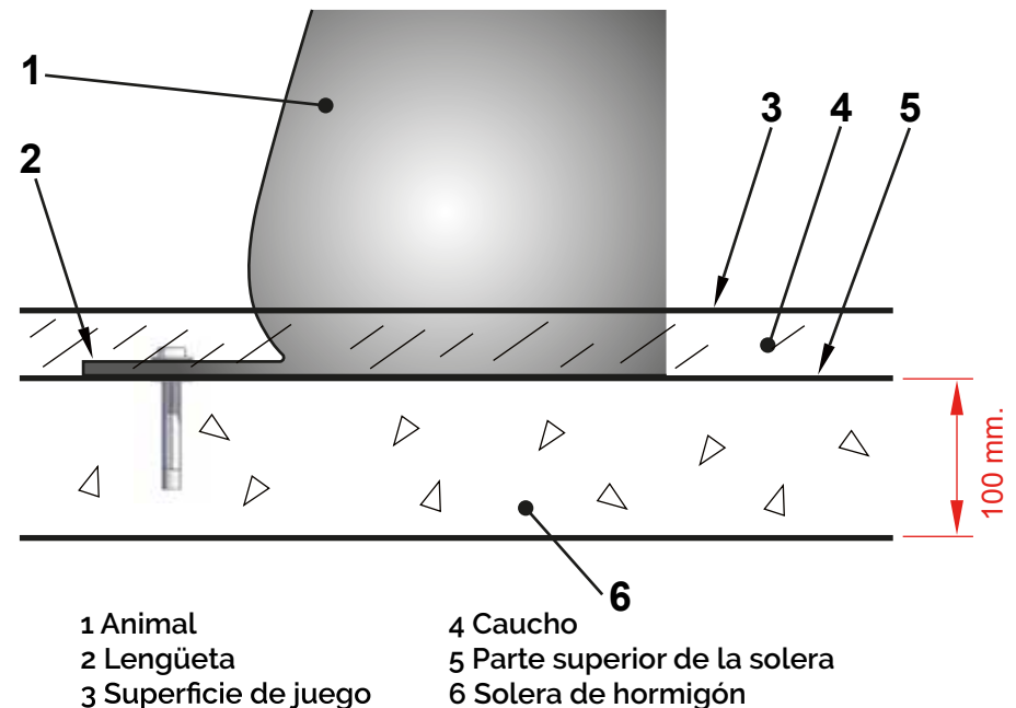
Detalle del anclaje
